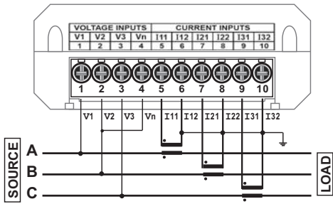
3CT(0~333mV)
