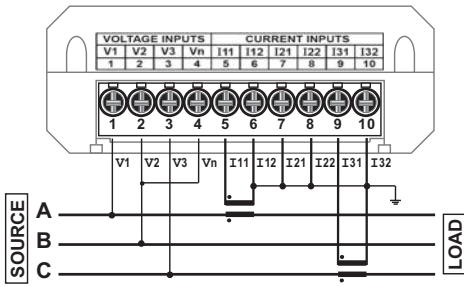
2CT(0~333mV)
